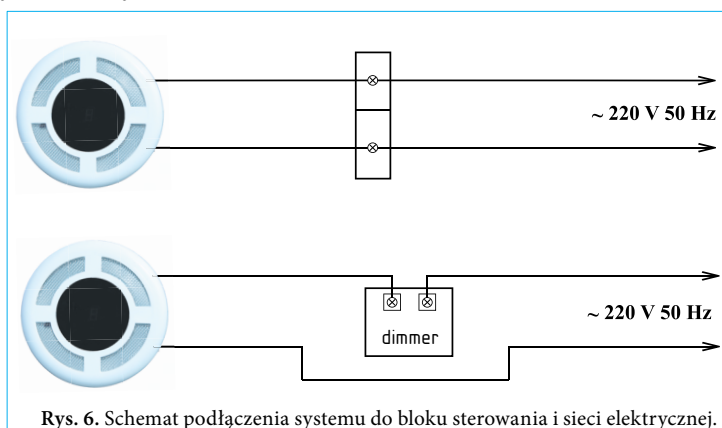
Rys. 6. Schemat podłączenia systemu do bloku sterowania i sieci elektrycznej.
