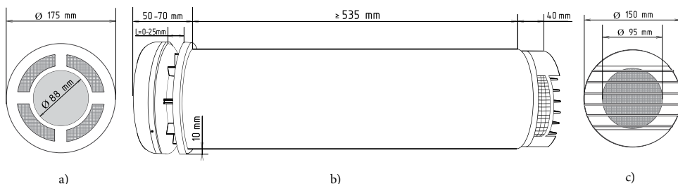
Rys. 2. Gabaryty i wymiary układu wentylacji PRANA-150: a) kratka wentylacyjna w domu; b) monoblok, cięcie wzdłużne; c) kratka wentylacyjna z ulicy.
