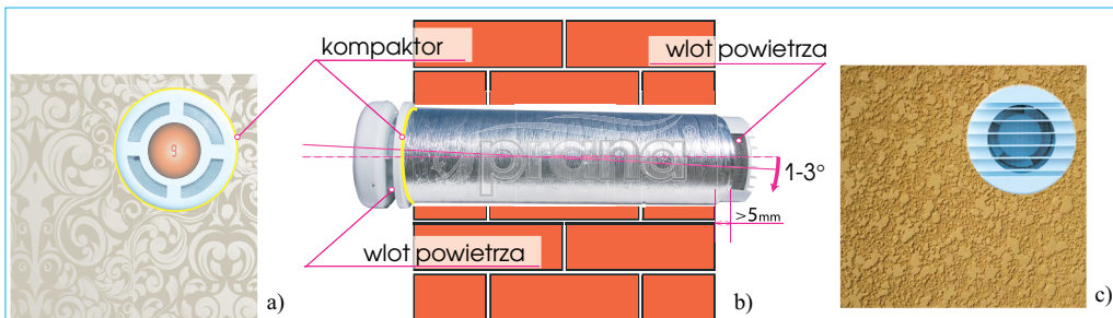
Rys 4. Schemat montowania układu wentylacji dolotowo-wyciągowej PRANA-150 w ścianie:
